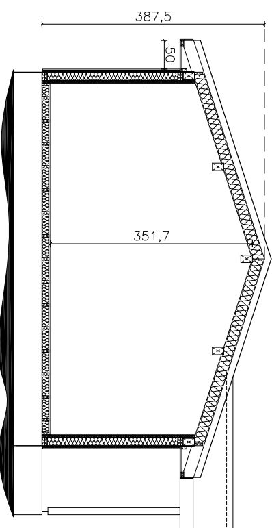
PRZEKRÓJ
